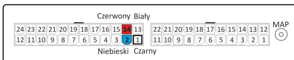
Widok od przodu sterownika EasyEcu 2
